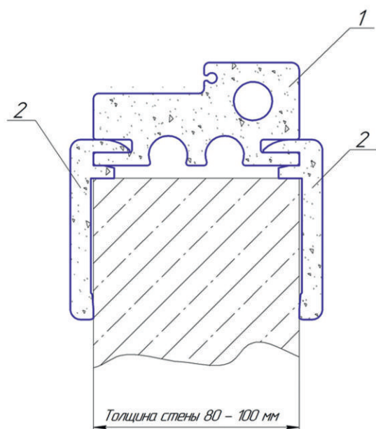
1 - Дверная коробка 80 мм 2 - Наличник F
