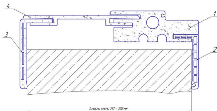
1 - Дверная коробка 100 мм 2 - Наличник L32 3 - Наличник L42 4 - Добор E150
