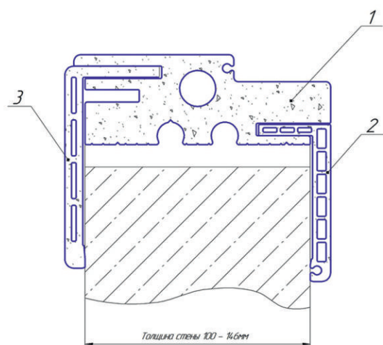
1 - Дверная коробка 80 мм 2 - Наличник F
