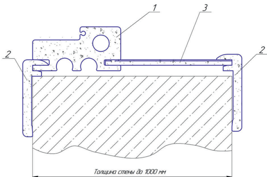
1 - Дверная коробка 80 мм 2 - Наличник F 3 - Добор прямой 5 мм
