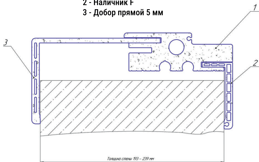
1 - Дверная коробка 100 мм 2 - Наличник L32 3 - Добор L135
