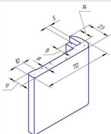
Добор телескопический L135
