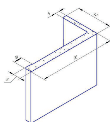
Добор телескопический E150 с двух сторон
