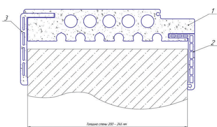
1 - Дверная коробка 200 мм 2 - Наличник L32 3 - Наличник L42
